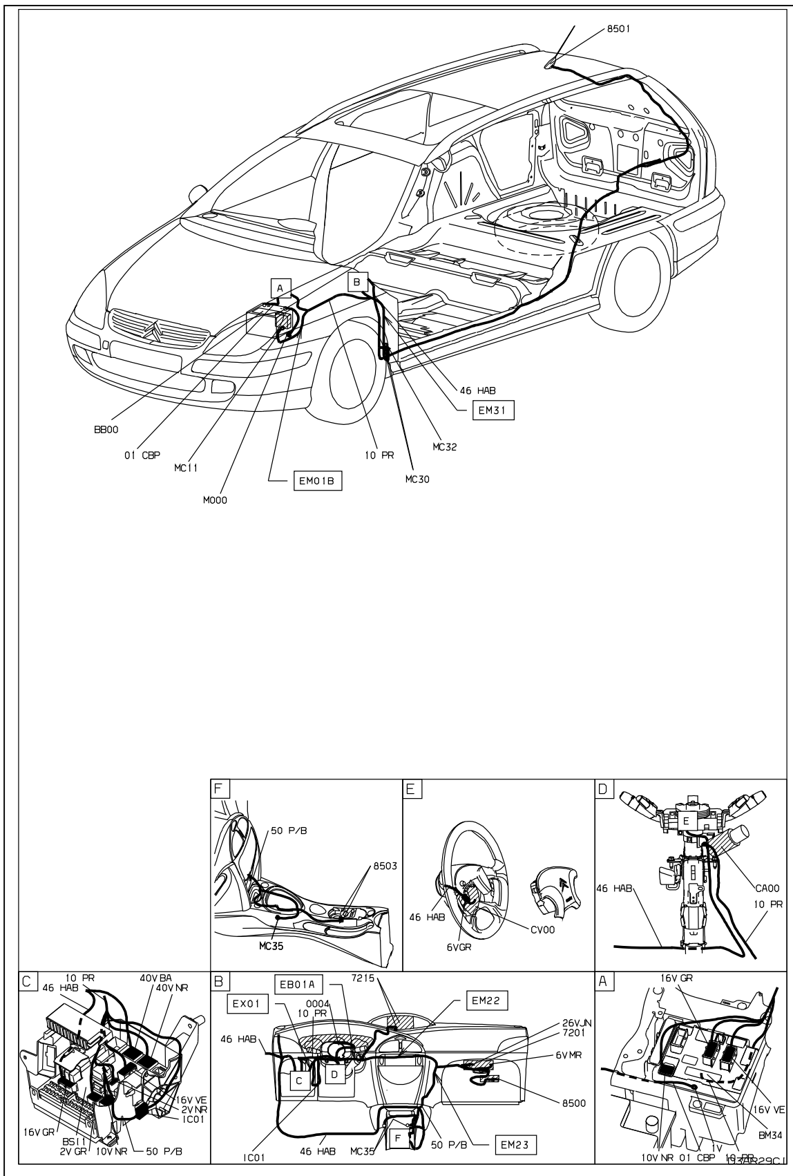
Schéma : D3AR29CI
