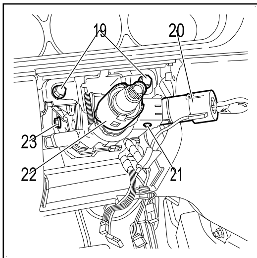
Schéma : C5EP129C
