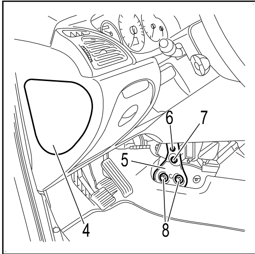
Schéma : C5FP0ARC
