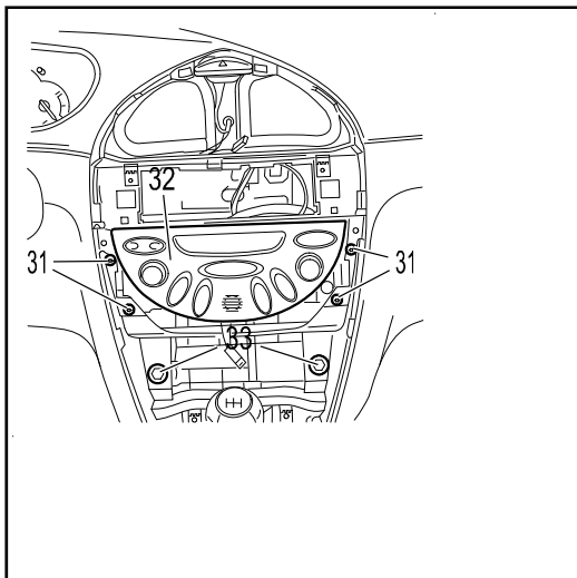
Schéma : C5FP0AXC
